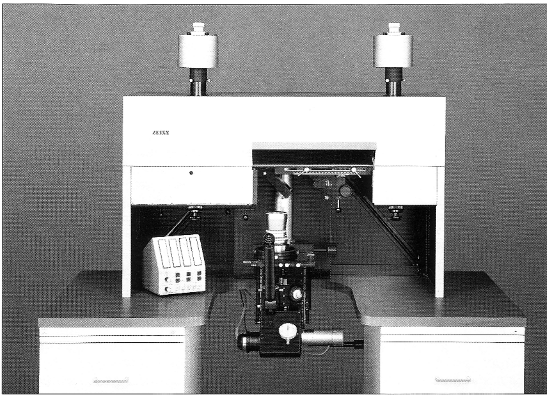
Abb. 6 Elektronisches Objektivprüfgerät K VI
