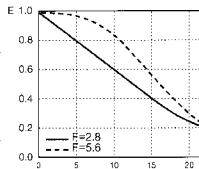
Relative Beleuchtungsstärke
