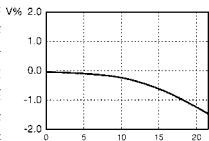
Verzeichnung in % der Bildhöhe
